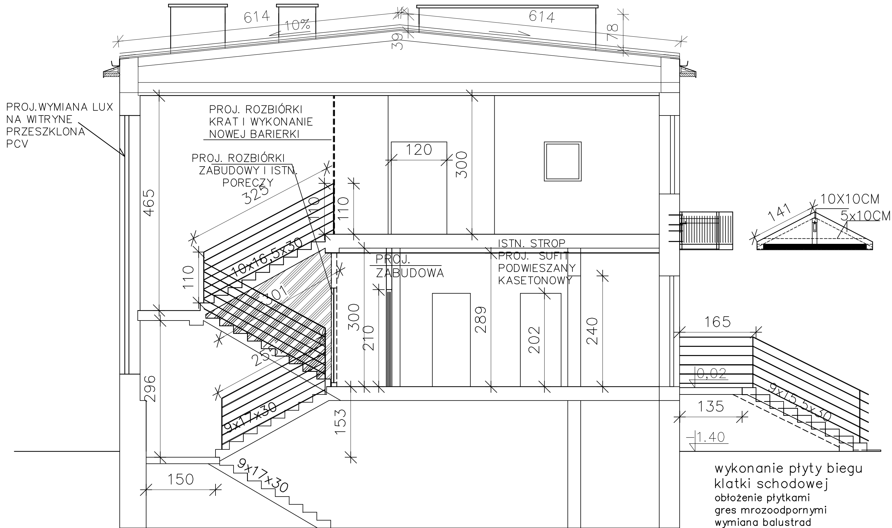
PRZEKRÓJ PIONOWY 1:50
