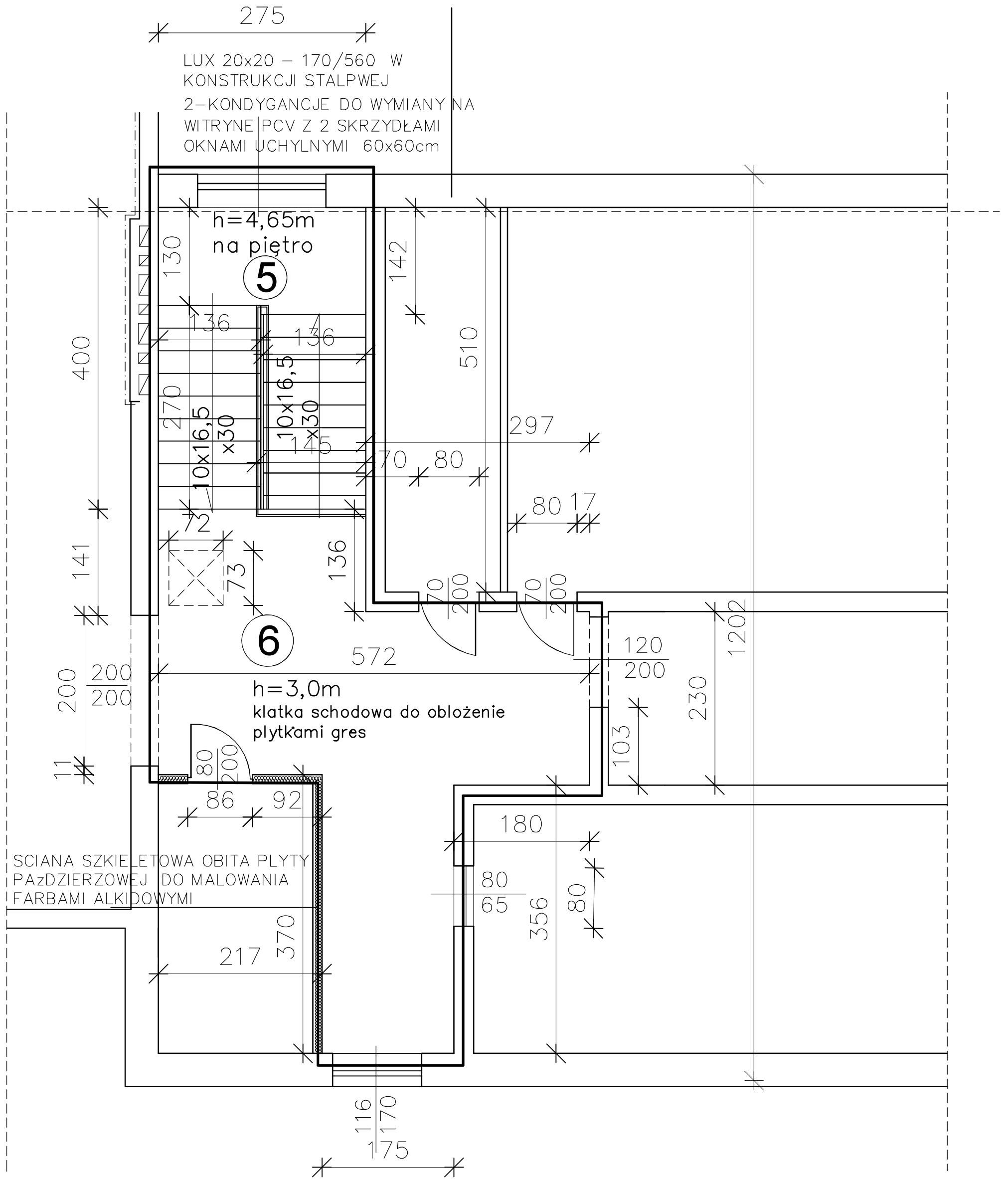
RZUT PIĘTRA 1:50
